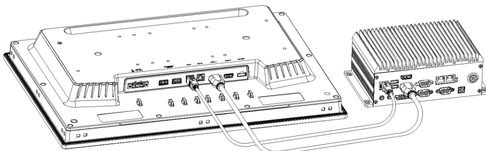
(HDMI 1 + USB 1 케이블 연결 구성)
